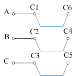
Монтажная
