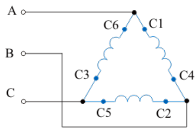
Принципиальная
